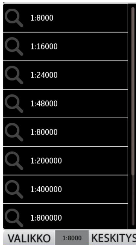
Kuva 6 Mittakaavan pikavalinta
