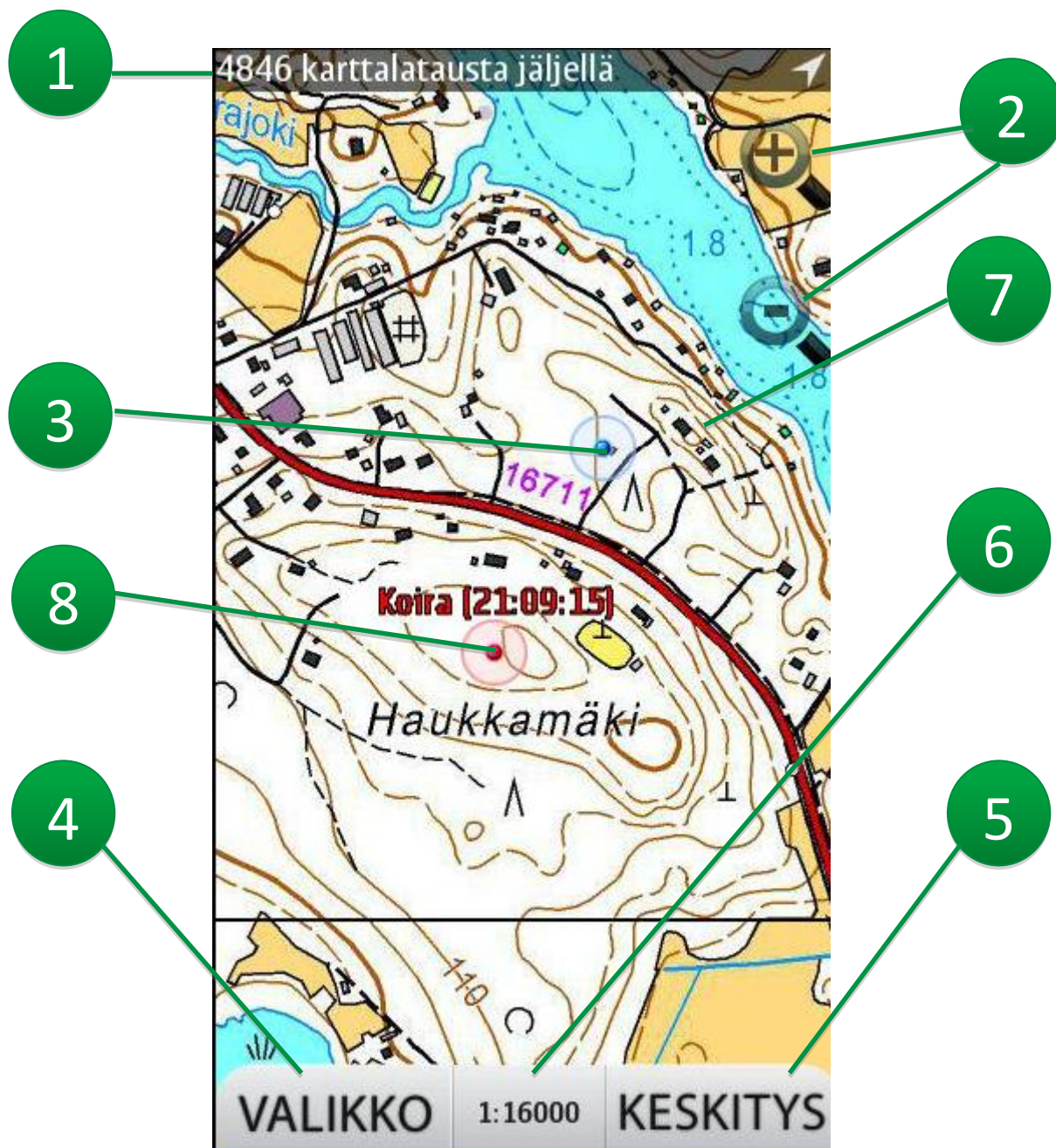
Kuva 1 Karttaselaimen päänäyttö
